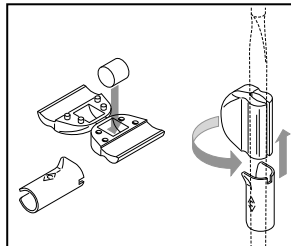
R1-023 Ghiera di chiusura corpo RL tipo Campagnolo Lockring for Campagnolo type FW body Ecrou pour corps RL type Campagnolo
