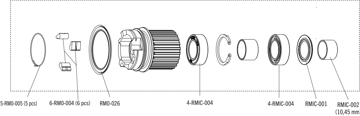
R0-127 (MICRO SPLINE 12 Ø33 mm ALU)
